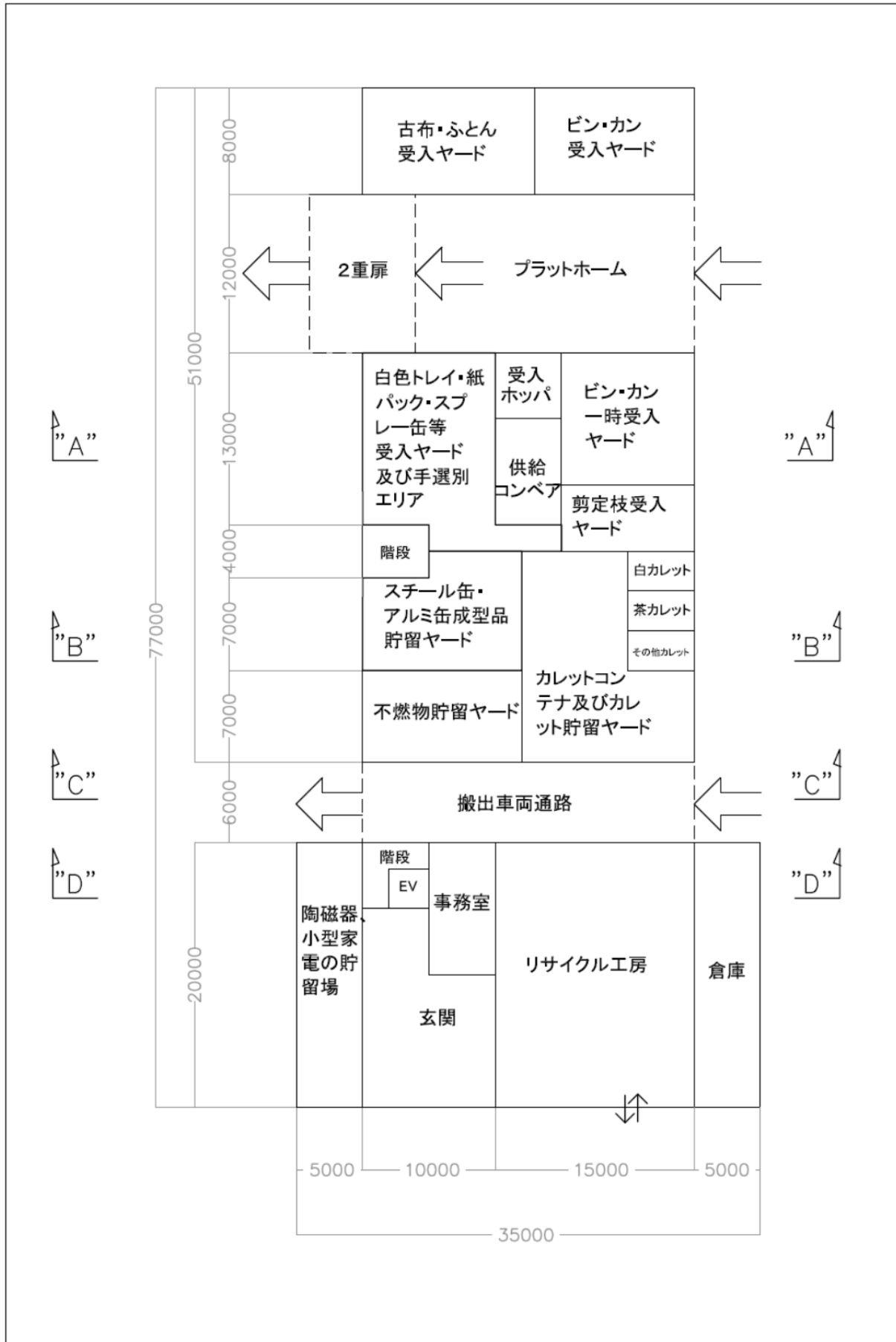
図8-1 1階平面計画図(案)
