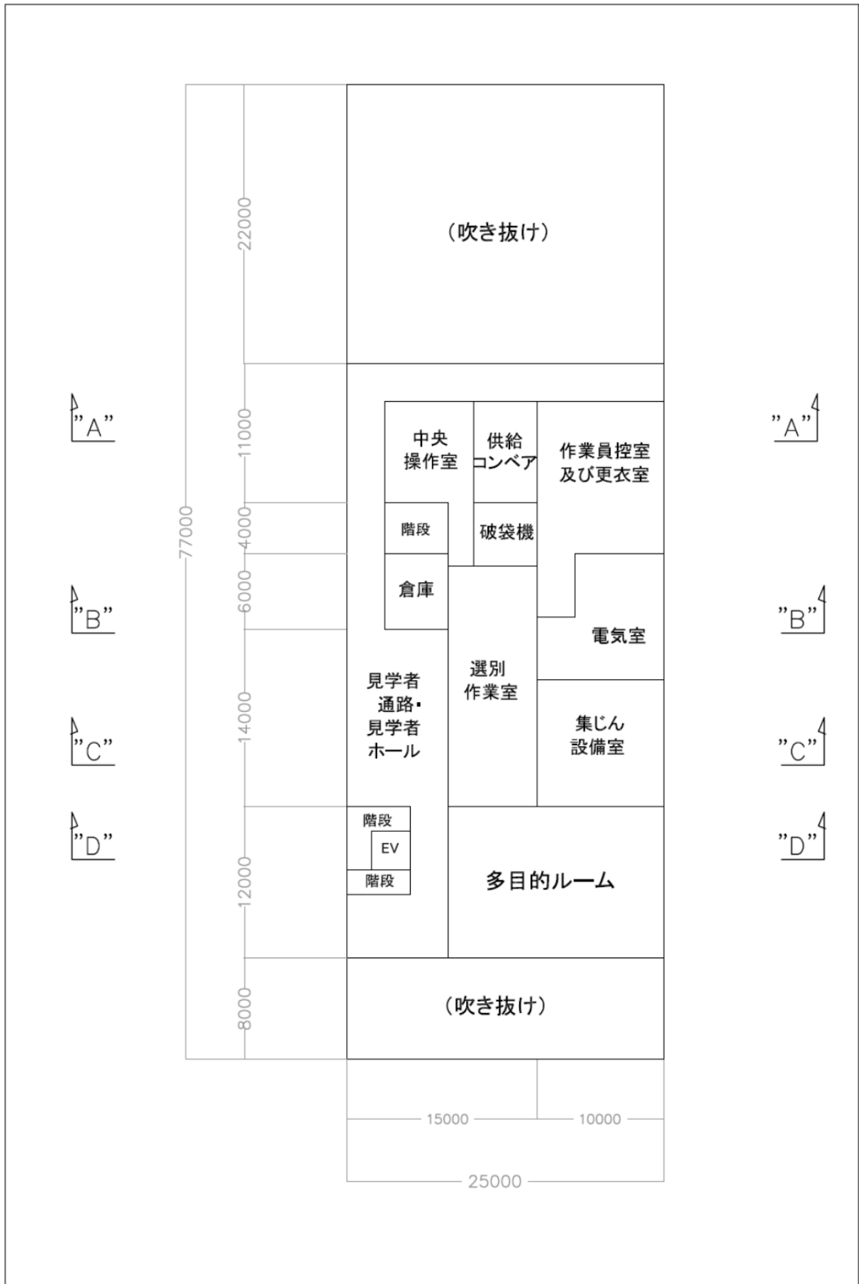
図 8-2 2 階平面計画図 (案)
