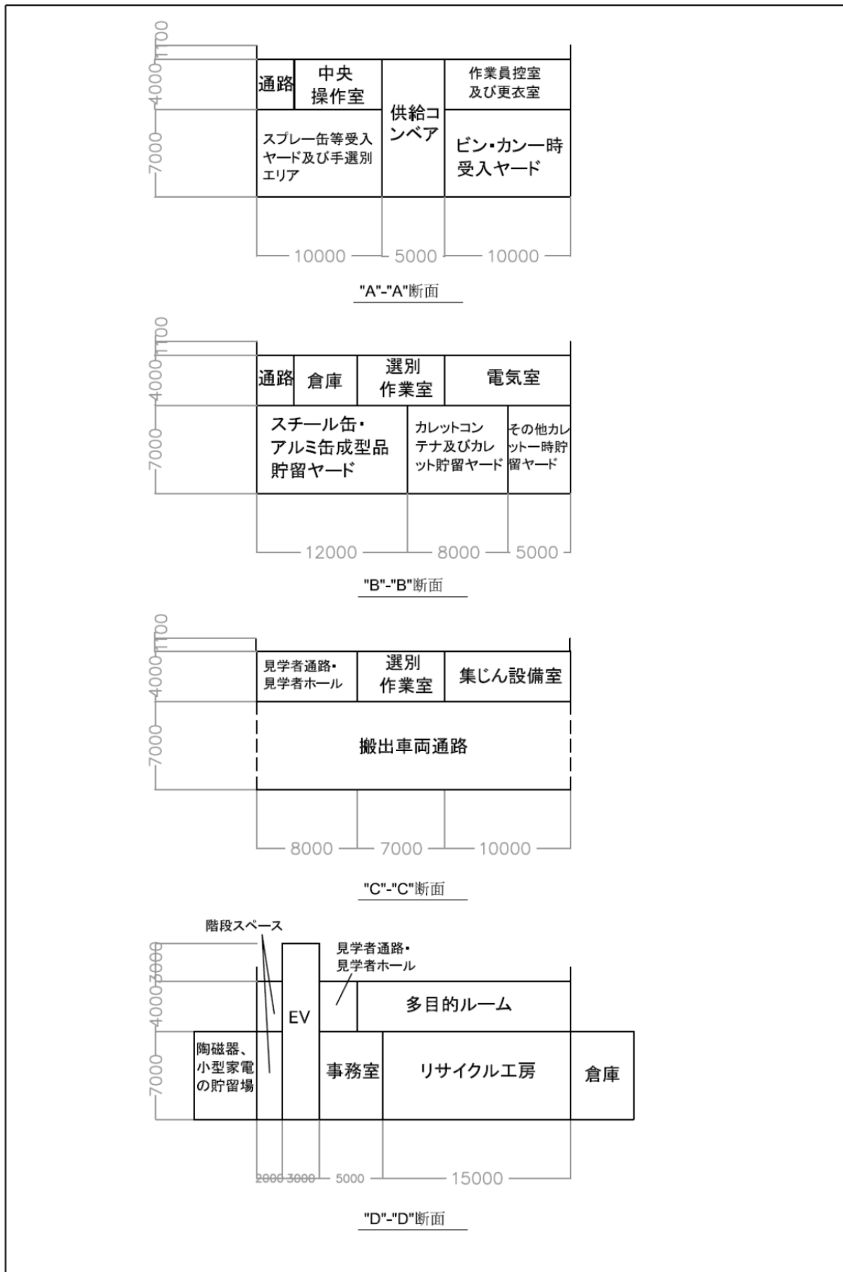
図 8-4 断面計画図 (案)
