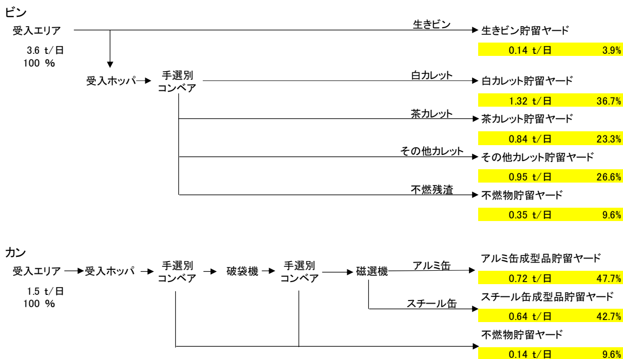
図4-1 ビン及びカンの物質収支図 (想定)
