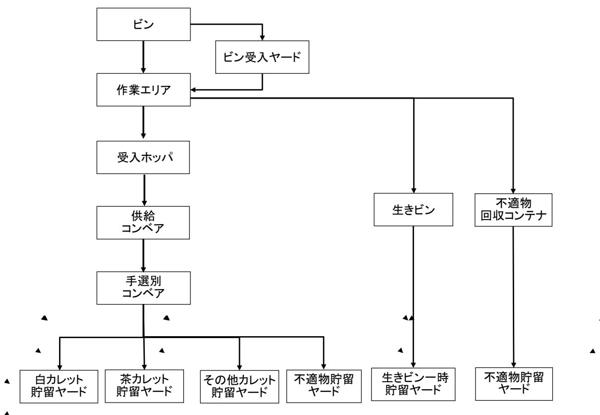
図3-1 ビンの基本処理フロー図
