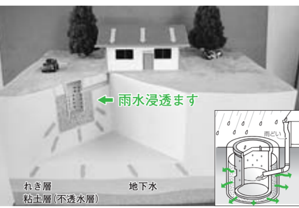
雨水浸透ますの模型
